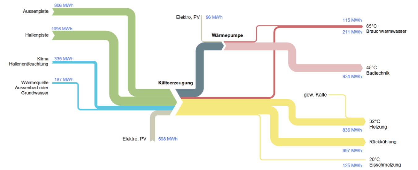
Jahres-Energieflussdiagramm
