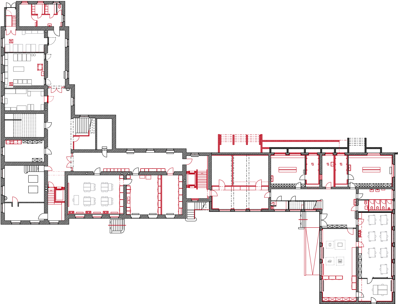
Grundriss Untergeschoss
