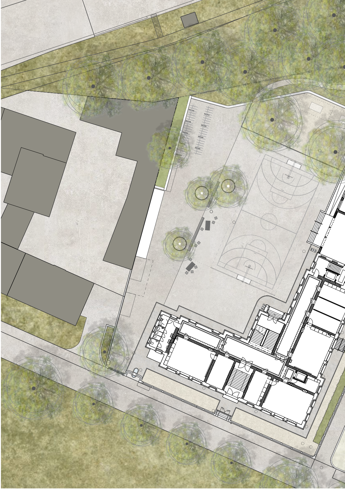
Umgebungsplan
