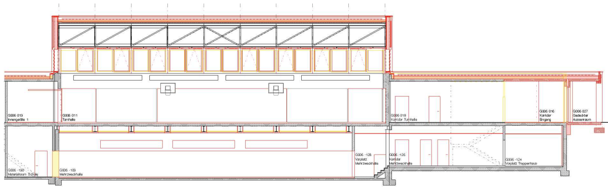
Längsschnitt Doppelturnhallegebäude
