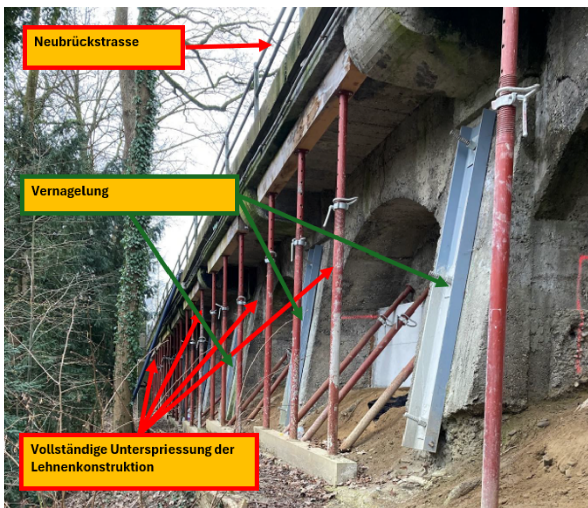
Abbildung 5: Bestehende Lehnkonstruktion inkl. der Sicherungsmassnahmen
