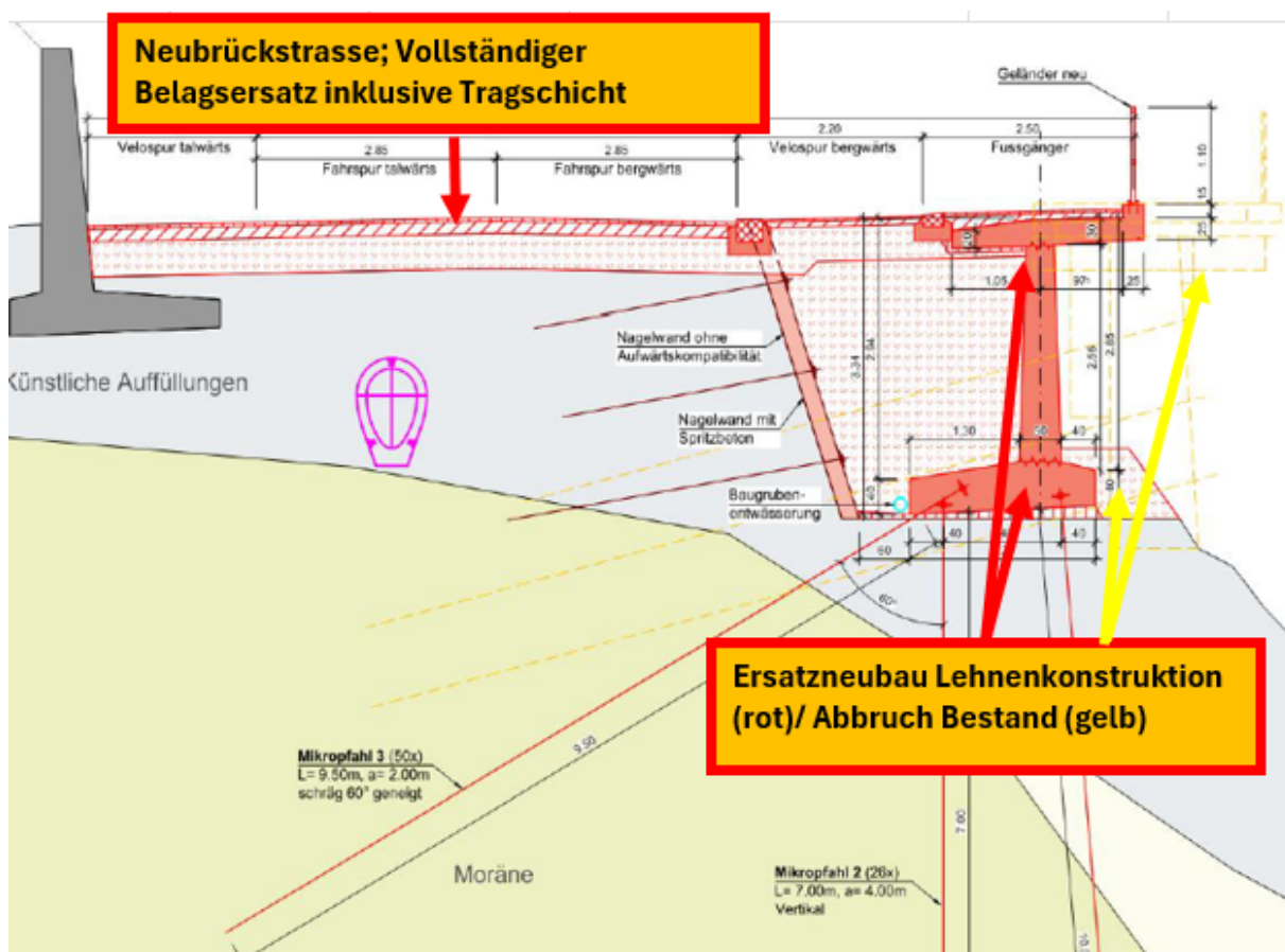
Abbildung 6: Geplanter Ersatzneubau
