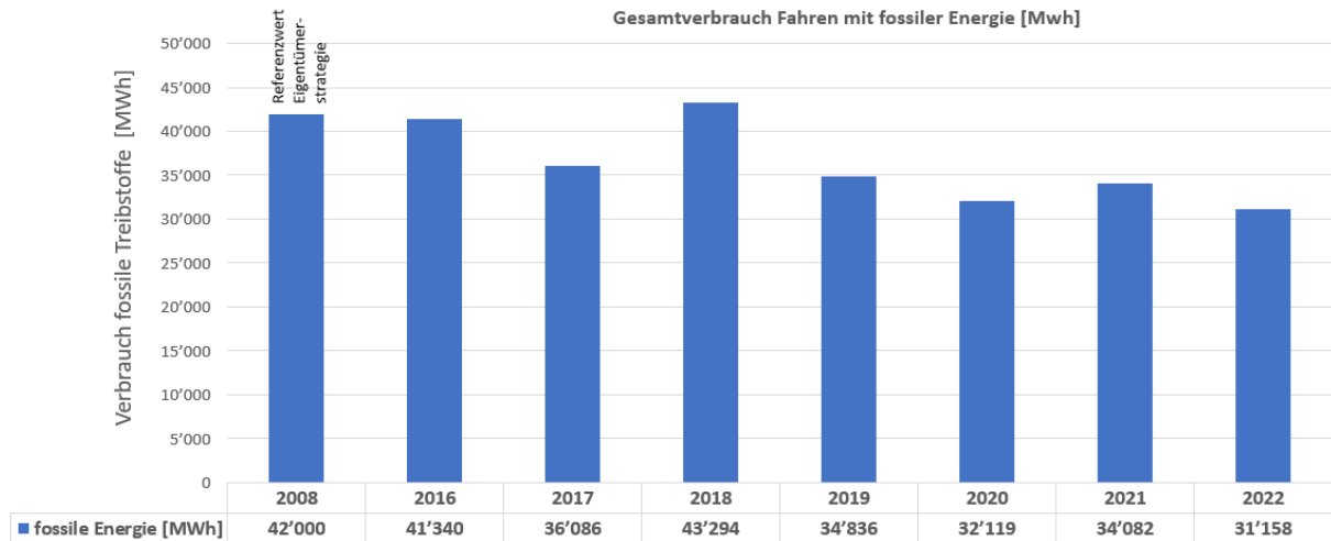
Abbildung 2: Fossiltreibstoffverbrauch 2016-2022 (Referenzjahr: 2008)
