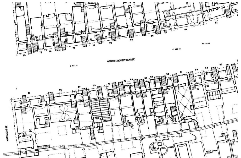
Abbildung 59: Ausschnitt aus dem Kellerplan der Unteren Altstadt Der Ausschnitt aus dem Bereich Kreuzgasse/Gerechtigkeitsgasse offenbart einerseits eine klare Typologie, andererseits eine überraschende Vielfalt von Formaten, Konstruktionsweisen und Erschliessungen der Keller
