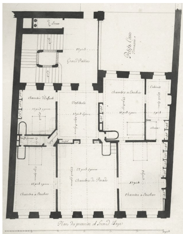
Abbildung 50: Gerechtigkeitsgasse 40, «Plan du premier et Second Etage», um 1730 (Planmappe PW159 der Burgerbibliothek).
