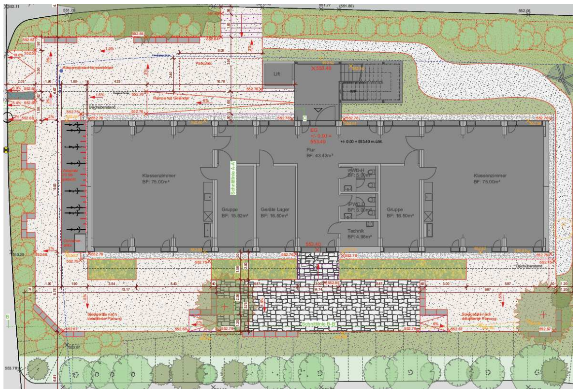
Abb.3: Situationsplan mit Umgebung
